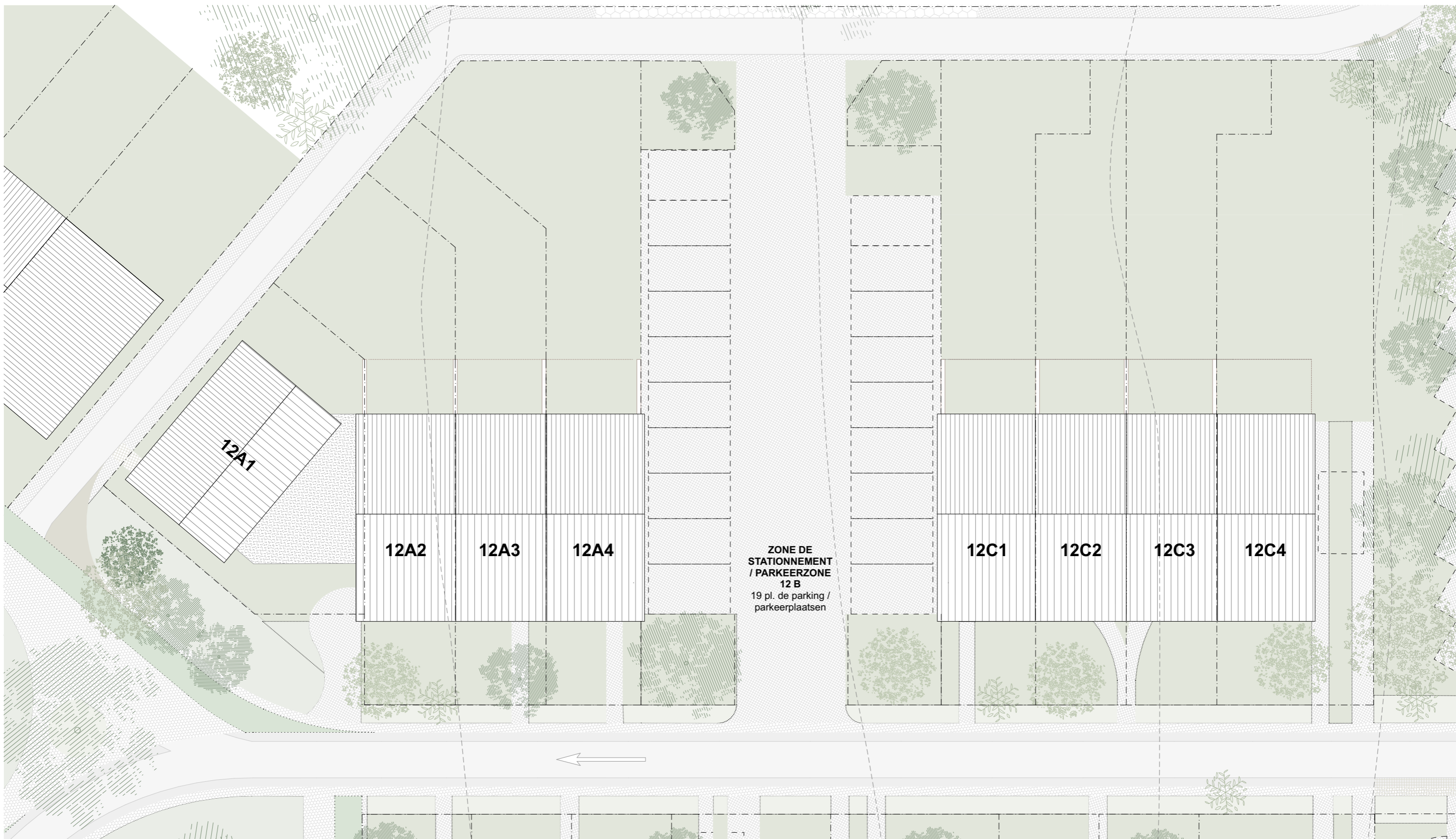
PLAN IMPLANTATION ZONE DE STATIONNEMENT - INPLANTINGSPLAN VAN DE PARKEERZONE 12B
